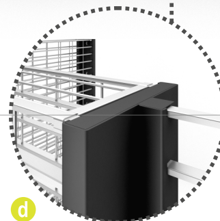
d POŁĄCZENIE Z PANELEM OGRODZENIOWYM SLIM CONNECTION WITH SLIM FENCING PANEL
