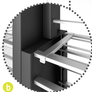
b POŁĄCZENIE Z PODMURÓWKĄ I PANELEM SLIM CONNECTION WITH BASE AND SLIM PANEL
